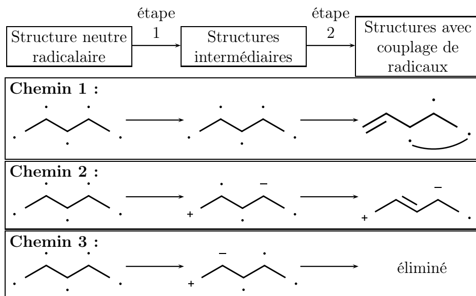
FIGURE 4.4 – Exemples de trois chemins qui génèrent des structures de Lewis localisées raisonnables pour la description de l'espèce radicalaire C_5H_7^\bullet . De cette manière, 39 structures peuvent être générées.
